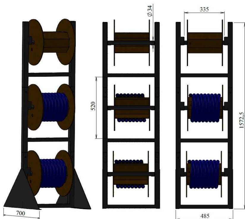
DÉTAILS PORTE-BOBINES POUR TUYAUX
