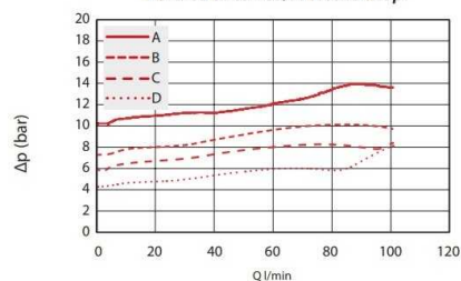
Perdite di carico/Pressure drop
