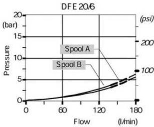
Pressure drop versus Flow P-> A(B) PERDIDA DE CARGA P-> A(B)
