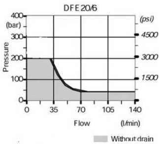
Pressure drop versus Flow P-> A(B) PERDIDA DE CARGA P-> A(B)
