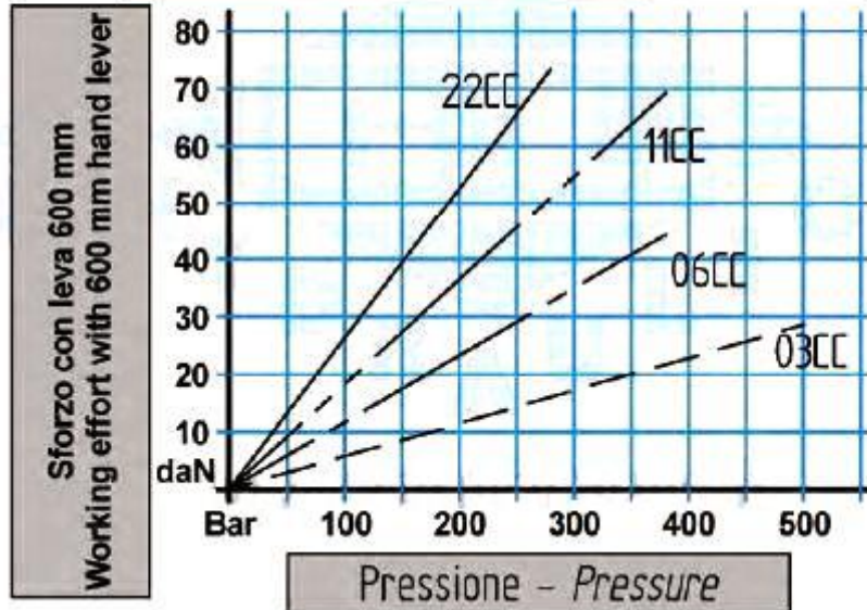
Diagramma prove di carico Load curve
