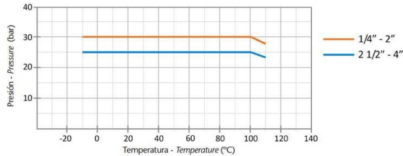
DIAGRAMA PRESIÓN - TEMPERATURA / PRESSURE - TEMPERATURE DIAGRAM
