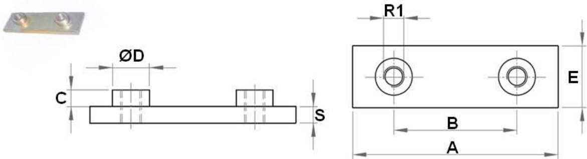
DIN 3015/2
