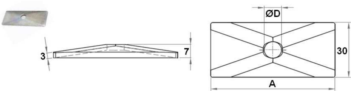
DIN 3015/3
