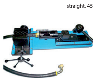
Introducción rápida para racores Manual nipple inserter
